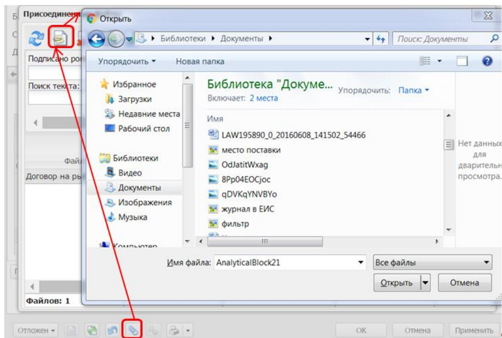
Рис. 20. Прикрепление документации
