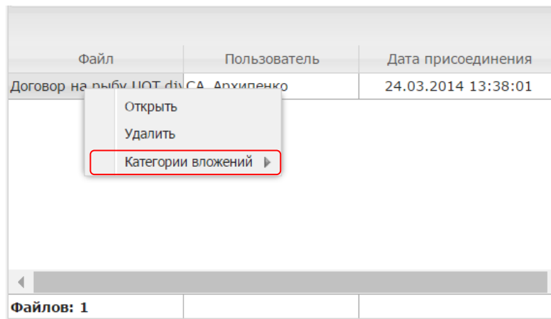
Рис. 21. Выбор категории
